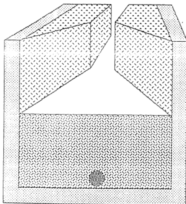
VISTA DE UNA SECCION ARQUETA - B
